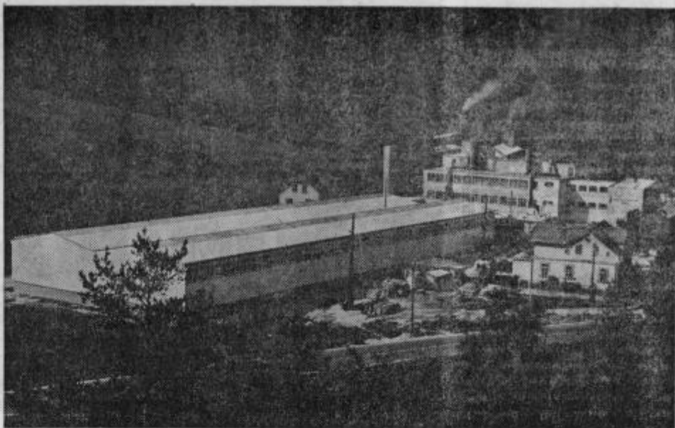
Nov del tovarne elektroporcelana v Izlakah, ki je bil cilj prve etape rekonstrukcije
