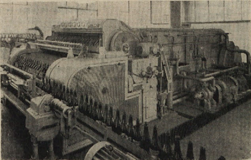
Avtomatična čistilnica steklenic brez krtač — Zmogljivost na uro: 7000 steklenic
