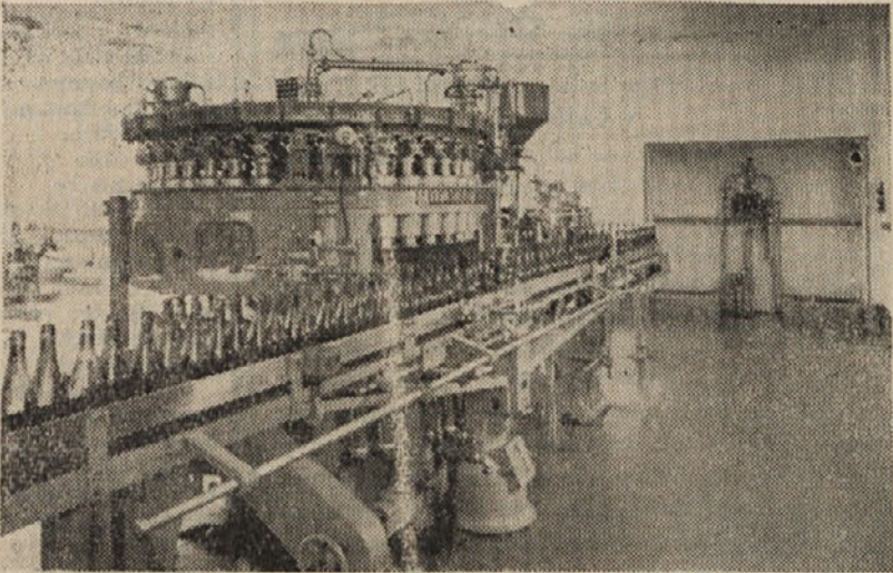
Stroj za polnjenje in zapiranje steklenic — Zmogljivost na uro: 7000 steklenic
