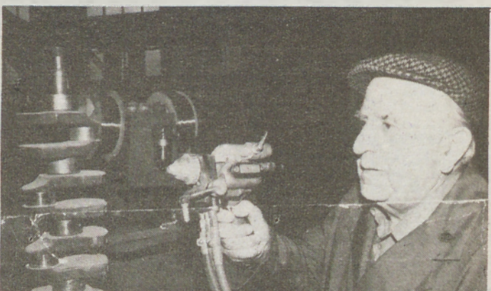
Izrabljena gred je zanič; ko pa nanjo nanesemo kovinske drobce in jo izstružimo, je kot nova. Na sliki Štefan Kofjač z eno od pištol za metalizacijo. Foto: J. Z.
