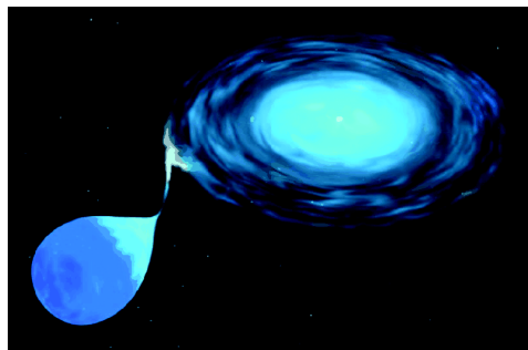
Hipotetičen prikaz, kako črna luknja požira bližnjo zvezdo
