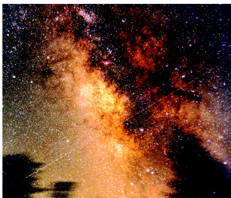
Jedro naše galaksije — Rimske ceste — zakriva ga velik oblak kozmičnega prahu
