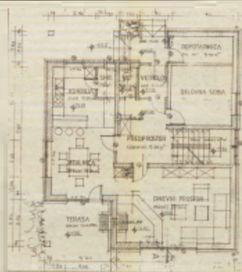
Tloris pritličja
