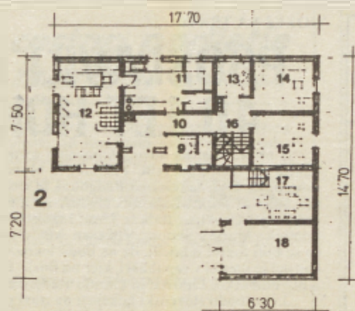
Tloris pritličja
