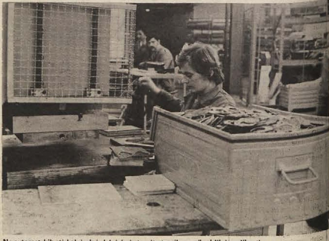
Na avtomatskih stiskalnicah izdelujejo iz tesnita tesnila raznih oblik in velikosti.
