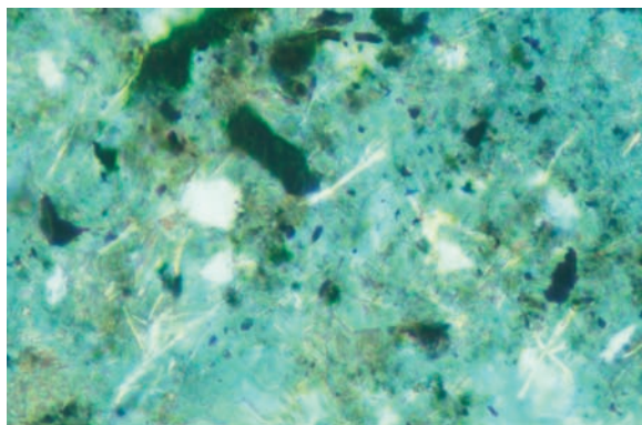
Sl. 3.3.5: Isto kot na sl. 3.3.4 . Pod navzkrižnimi polarizatorji so lepo vidna večja kremenova zrna (belo). Sivo so drobna večinoma kremenova zrna, med katerimi so večja in manjša neprozorna zrna in podolgovati preseki iglic rutila in lističev sericita, ki imajo visoke interferenčne barve (rumenkasto). Presevna polarizirana svetloba, + N, dolžina dolgega roba slike 0,14 mm.
