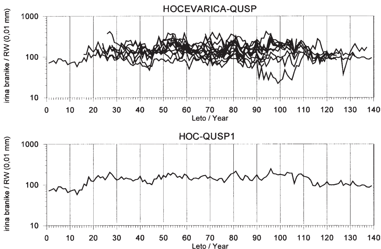
Sl. 6.2.4: Zaporedja širin branik sinhroniziranih hrastovih vzorcev (zgoraj) in plavajoča kronologija HOC-QUSP1 dolga 139 let (spodaj). Na abscisi so prikazana relativna leta.
