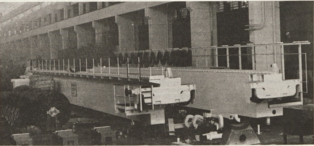
80-tonski žerjav za TOZD PUM v fazi montaže (Foto: E. L.)
