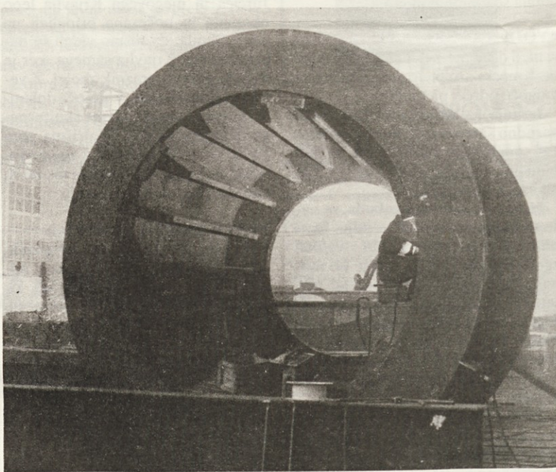
Podstavek ležaja za HE Haditho v fazi varjenja (Foto: E. L.)
