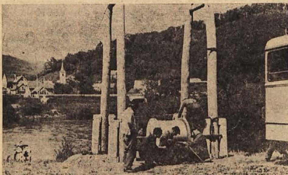
ELEKTRO CELJE – POSLOVNA ENOTA KRŠKO gradi v spodnjem delu Sevnice novo transformatorsko postajo, ki jo kraj nujno potrebuje. – Na sliki: delavci pri gradnji daljnovoda čez Savo. (Foto: Franc Pavkovič)
