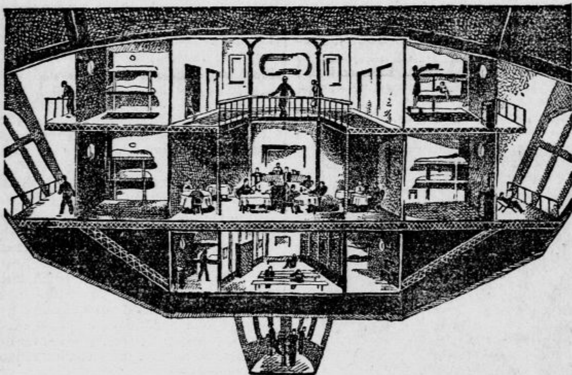
Notranjščina potniškega zrakoplova »R 100«.
