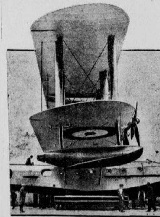
Največji mornariški letalni čoln so dovršili na Angleškem. Čoln je ves iz duraluminja, ima tri motorje s skupno nad 2000 k. s. in akcijski radij 2400 km.
