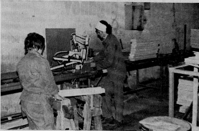
Nabijanje sidrinih letvic na podboj
