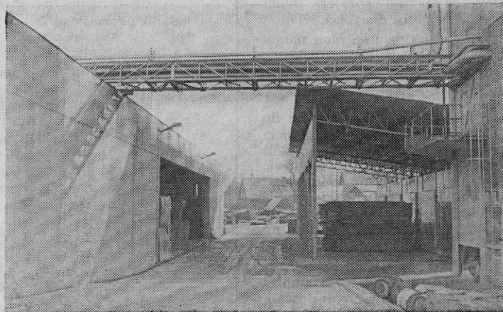
Na sliki je desno del kotlovnice s sušilnimi komorami, levo pa skladišni prostor umetno sušenega lesa in drugih materialov. Od zgoraj je sistem cev, ki vodijo po eni strani skoblance in žagovino v kotlovnico, kjer izgoreva. V sklopu sistema pa se po ceveh vrača potrebna energija za sušenje lesa in ogrevanje prostorov v TOZD Rečica
