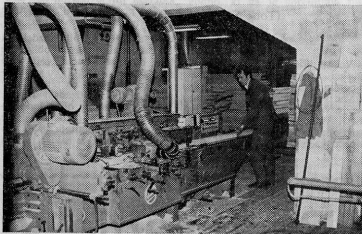
»Gorjana« — večstranski skobelni stroj, skobljanje podboja
