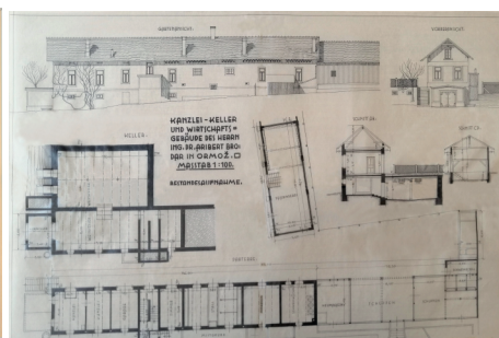
Načrt za vinsko klet ob Brodarjevi vili iz leta 1939. Hrani: Zgodovinski arhiv Ptuj.
