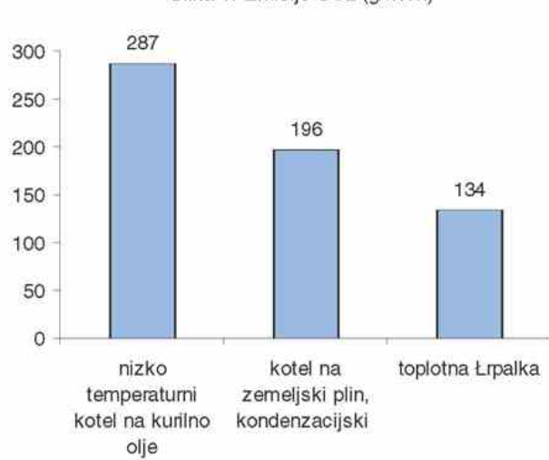
Slika 1: Emisije CO 2 (g/kWh)
