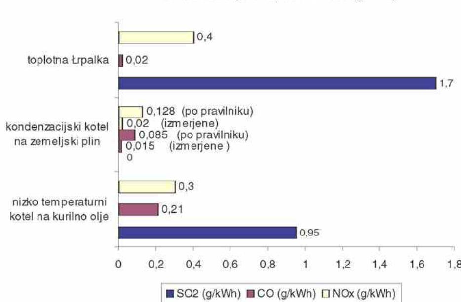
Slika 2: Emisije SO 2 , CO in NOx v (g/kWh)
