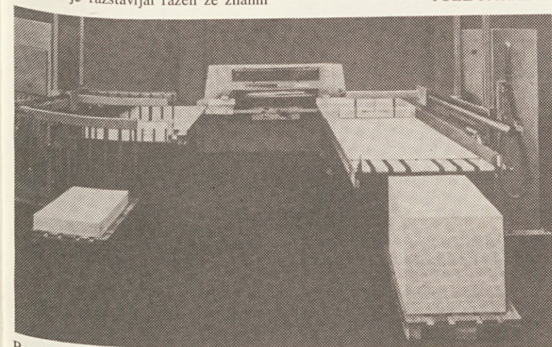
Rezalni stroj Wohlenberg z vlagalno in izlagalno mizo
