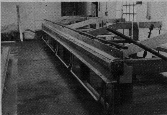
Kovinski delavci Komunalnega podjetja so si pomagali, ko so sami naredili stroj za krivljenje pločevine večjih razsežnosti. Tako so prihranili drago prevažanje pločevine v Celje, sedaj lahko ta dela opravijo kar doma.
