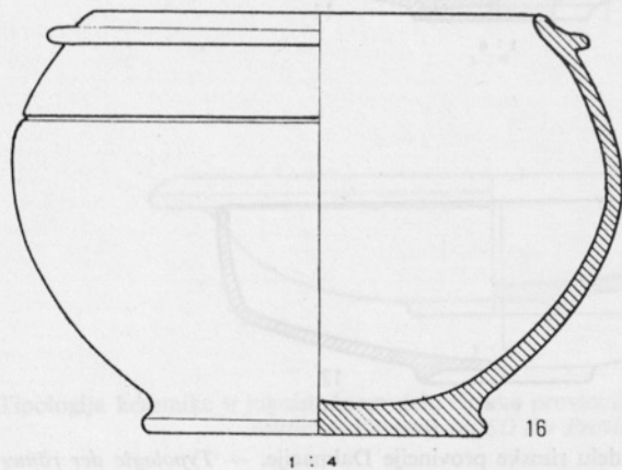
4 Tipologija keramike u jugoistočnom delu rimske provincije Dalmacije. — Typologie der römisch-zeitlichen Keramik im SO der Provinz Dalmatien
