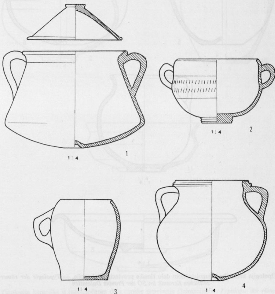
1 Tipologija keramike u jugoistočnom delu rimske provincije Dalmacije. — Typologie der römischzeitlichen Keramik im SO der Provinz Dalmatien
