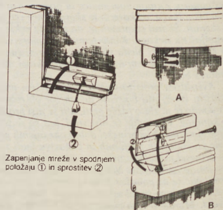
Prikaz bočne pritrditve KOMARNIKA P (A) in zaskočne pritrditve KOMARNIKA R (B)
