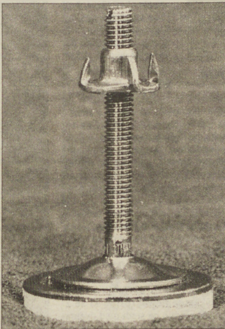
Nastavitveni vijak Staneta Tkalčiča, ki bo poenostavil in izboljšal polaganje lesenih podov in parketov.
