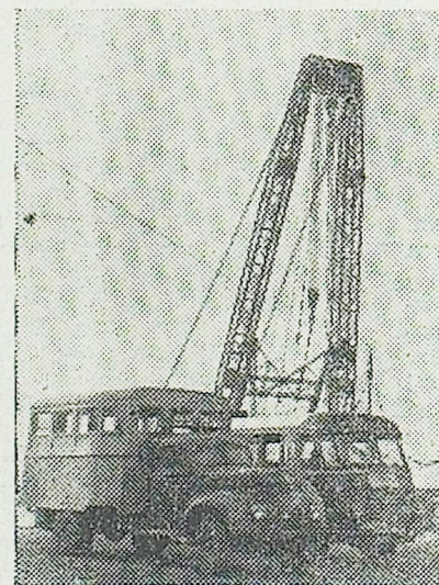
Za prevoz po suhem in morskem velikan za dvigovanje potopljenih delov ladij.
