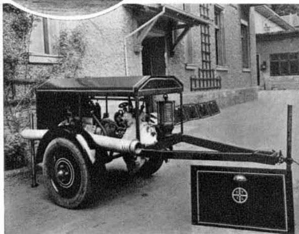
Motorne brizgalne, ki jih izdelujejo Strojne tovarne in livarne v Ljubljani.
