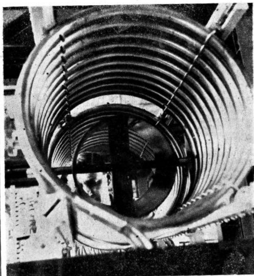
Ne vodovodna cev — već unutrašnjost jednog kruga za štimovanje jedne kratkotalasne stanice
