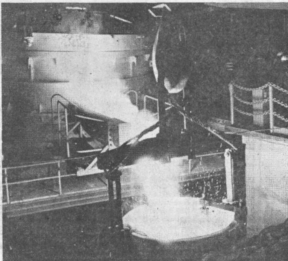
Velika delovna zmagaja: v Litostroju je steklo jeklo iz nove 25-tonske elektro obločne peči
