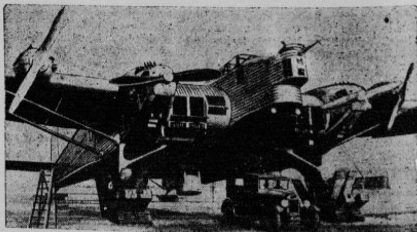
»Letišča trdnjave«. Francoska armada je dobila najnovejši tip letal, ki jih, vsled njihove konstrukcije imenujejo »leteče trdnjave«. Letalo je dolgo 21 m, široko 37 m in doseže hitrost do 200 km na ur. Oboroženo je z devetimi strojnimi puškami in prevaža lahko 2500 kg bomb.
