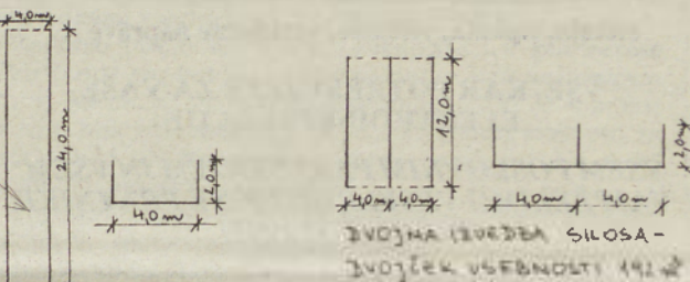
Skica 3: Dve različni izvedbi prevoznega koritastega silosa vsebnosti 192 m³
