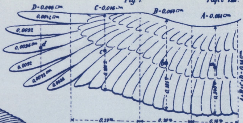
Flügel eines 4 kg schweren Storches Maßstab 1/4 natürlicher Größe
