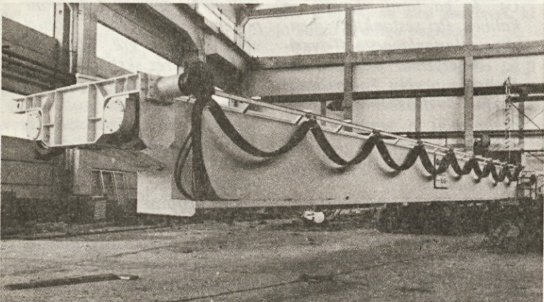
Mostno dvigalo z zmogljivostjo 50/16 ton je bilo izdelano za čistilnico nove livarne. Dolgo je 22 m in pripravljeno za transport (Foto: E. L.)
