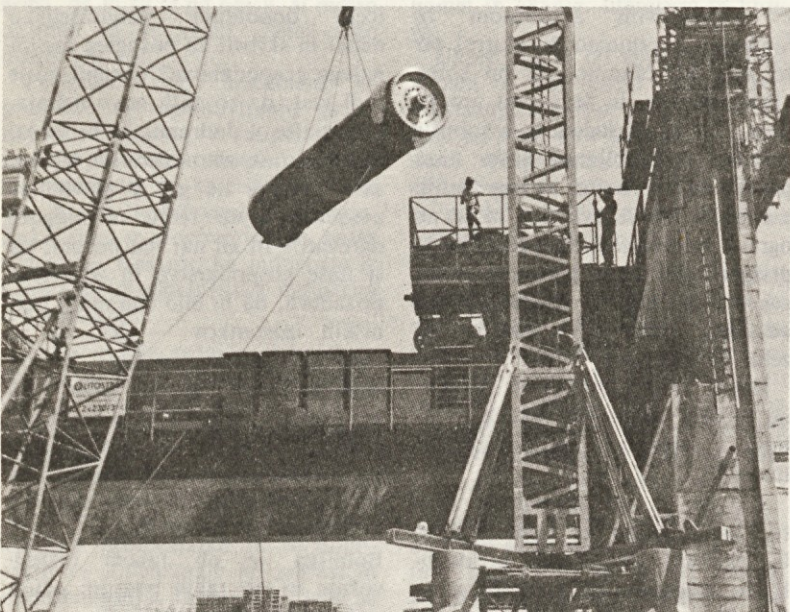
Boben glavnega dviga v montažnem postopku
