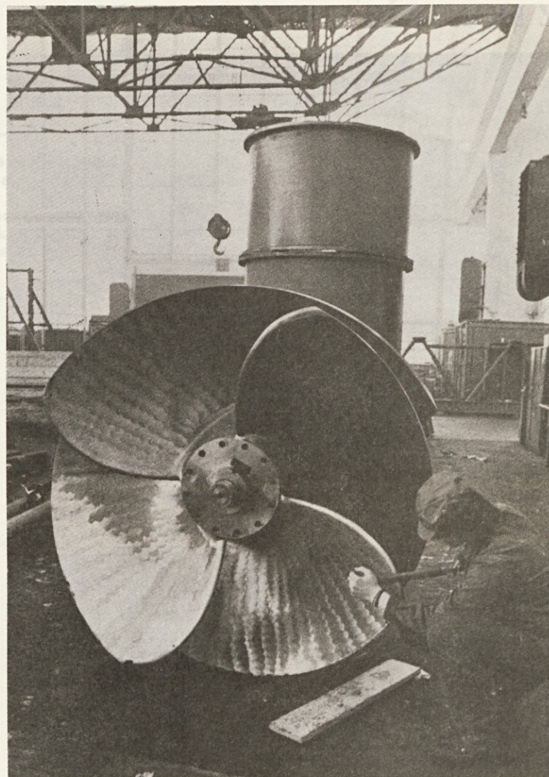
Rotor vijačne črpalke — VI 4,2/175 za hladilno vodo TE OBRENOVAC »B«. Višina črpanja H = 16,4 m, Q = 10,4 m pri N = 297 o/min. (Foto: E. L.)
