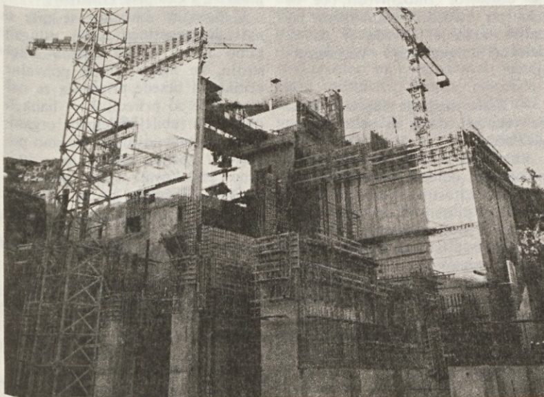
Pogled na dvigalo in odprto strojnico iz odtočne smeri. Dvigalo, z največjo zmogljivostjo, kar smo jih v Litostroju naredili, se kar izgubi na gigantskem gradbišču bodoče hidroelektrarne.
