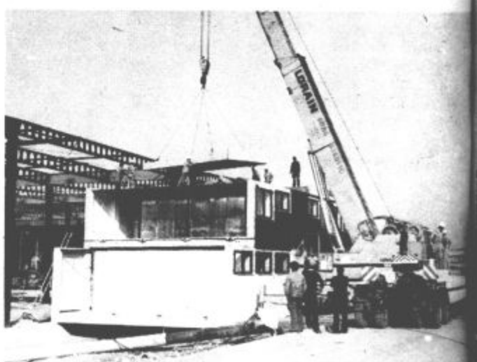
S prostorskimi elementi je GIP Vegrad Velenje gradil tudi prizid k novemu obratu tozda Zamrzovalniki TGO Gorenje Velenje
