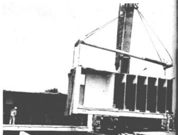
Montaža prostorskih elementov, celic, ki jih izdelujejo v tovarni pri Velenju
