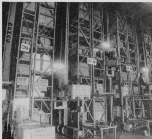
Vskladiščenje blaga za široko potrošnjo v regalnem sistemu v skladišču Bukovžlak.
