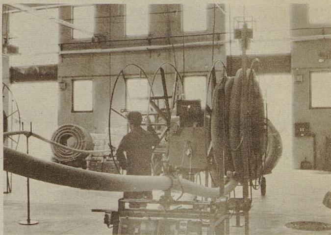
Proizvodnja drenažnih cevi na Ložnici.
