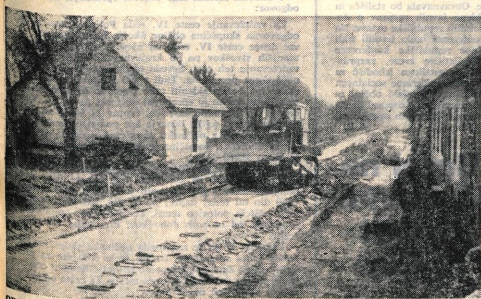
OBNOVA CESTE ZABNICA—ZGORNJE BITNJE — Cestno podjetje Kranj je pred nedavnim začelo obnavljati odsek ceste med Zabnico in Zgornjim Bitnjem. Ta cestni odsek bo približno 1,5 metra širši od lani obnovljenega cestnega odseka Škofja Loka—Zabnica. Letos namerava jo na obnovljeni odsek položiti bitogramoz, spomladi pa še asfaltbeton. Obnovljeni odsek bo dolg okrog dva kilometra. — A. Z. — Foto: F. Perdan
