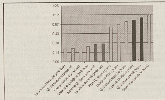
Povprečni razmik v času (ura : minuta) med odhodi vozil na obravnavanih relacijah
