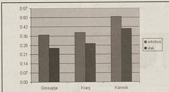
Slika 2: Primerjava med povprečnim časom potovanja in povprečno hitrostjo potovanja različnih prevoznih sredstev na obravnavanih relacijah.
