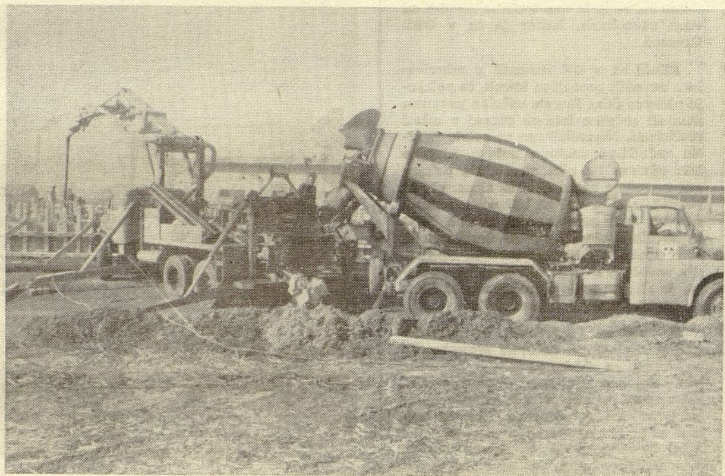
Gradis gradi nasproti železniške postaje Žalec poleg TOZD Strojna temelje za velike silose TOZD Mešalnica, ki se bo ob silosih razvila v nov in velik obrat.
