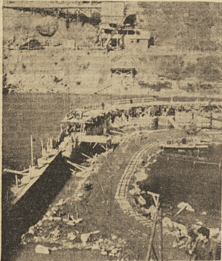
Cez nekaj mesecev je rebrasta betonska zagatna stena že varovala delavce pred valovi. — Do maja letos so gradbinci na Vuhredu izkopali iz gradbene jame nad 60.000 kubičnih metrov zemlje
