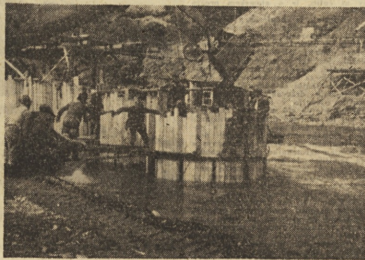
Tesarji so opazili zagatno steno meter za metrom, betonirni pa so jim bili z betonom vedno za petami. Tako se ponavlja v Vuhredu tekma med tesarji in betonirni dan za dnev
