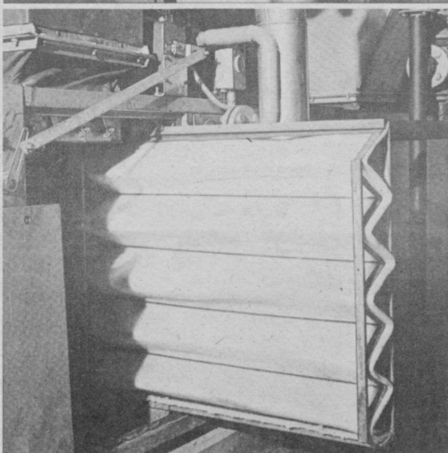
Dva izmed KOFIL – filtrov za čiščenje zraka, ki jih v Konusu izdelujejo v ploščah različnih dimenzij. KOFIL je netkani material izdelan iz sintetičnih vlaken, kemično ojačan z umetnimi smolami, zato pri uporabi skoraj nič ne menja svoje strukture.
