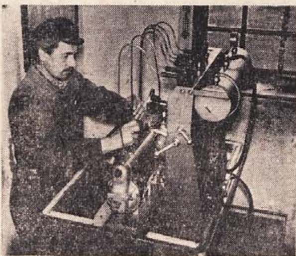
Jože Rajh, avtomehaničar iz mehanične delavnice »GORJANCI« v Straži: ob sodobnem stroju za preizkušanje tlačilk ugotavlja, ali so te še v redu. Tudi tak stroj sodi med sodobno opremo, kakršne ni najti v vsaki delavnici
