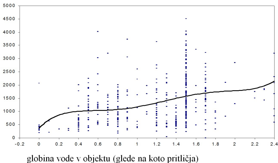
Graf 2: Krivulja poplavne škode, izdelana na podlagi ovrednotenih podatkov popisane poplavne škode (vir URSZR) za 454 enostanovanjskih hiš v poplavi leta 1990 (Celje, Medlog).
