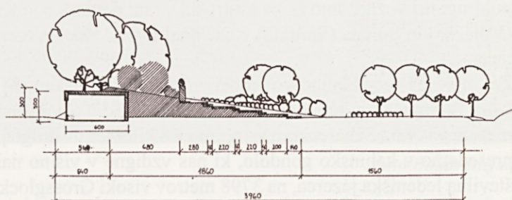
PREREZ A-A
