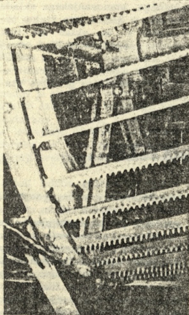
Konični boben Panzove žičnice 1972 - foto Veber
