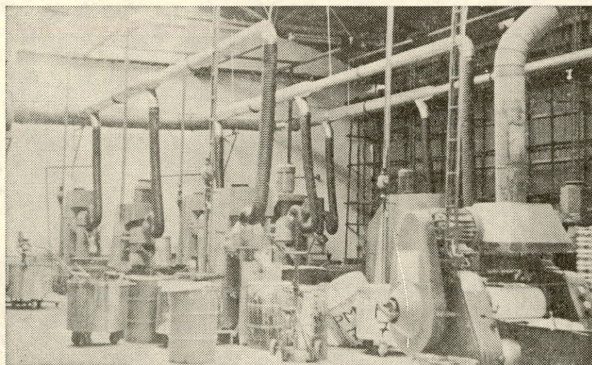
Pogled na novo ventilacijo v ribalnici...
