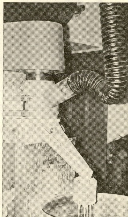
Premična odsesovalna havba pri peščenem mlinu...
