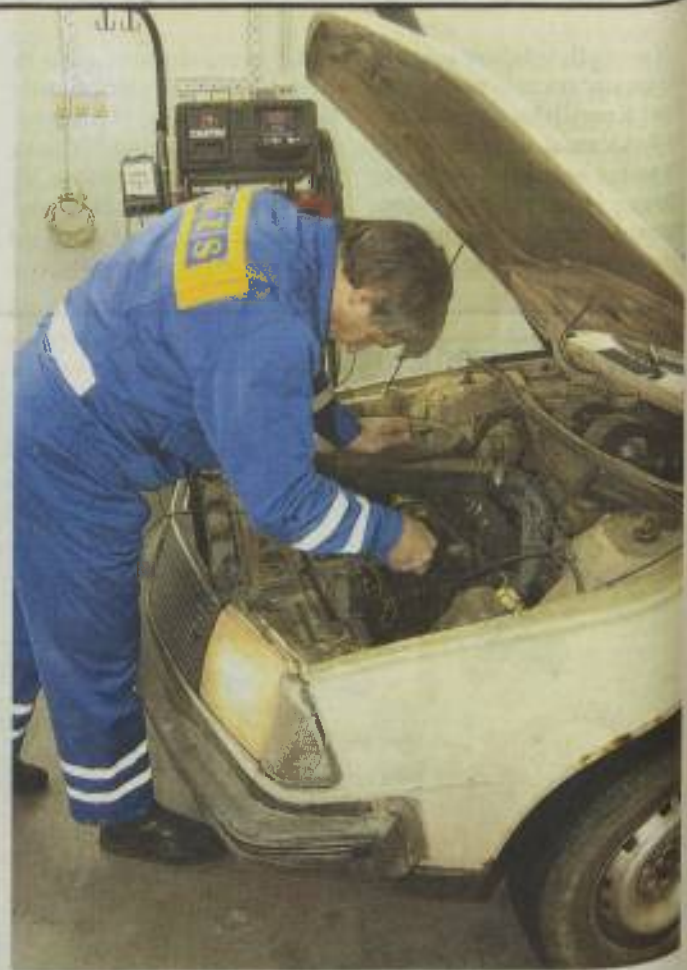
Pri meritvi emisije izpušnih plinov namestijo na vozilo senzorje za meritve temperature motorja in senzorje za meritve vrtilne hitrosti.
