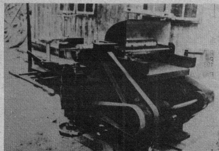
Skobelni stroj, izdelek mojstra Martina Marolta z Ljubnega
