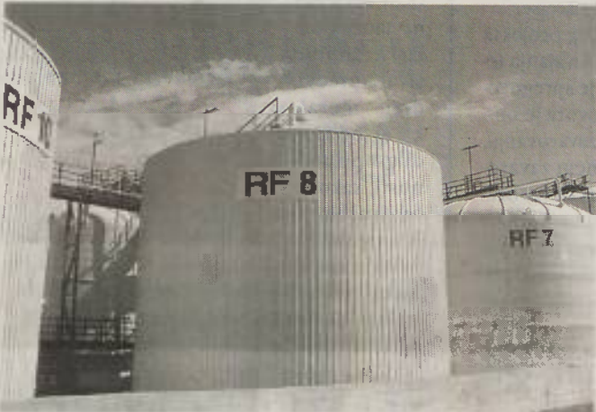
Rezervoar RF 8 je za Luko Koper zgradila Nafta Strojna, njegove karakteristike pa so volumen 750 kubičnih metrov, premer 11 metrov, višina 8,2 metra, hrupavost <0,8 µm ter gretje na dnu in pod plaščem rezervoarja.
