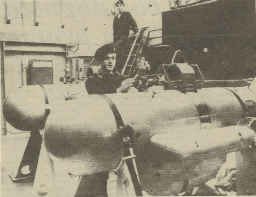
Plovec na britanskem minolovcu z vgrajenim generatorjem, ki sprošča magnetno polje in posnema šume ladijskih vijakov (Telefoto AP)
