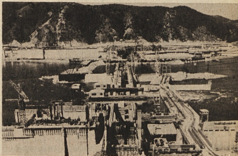
Pogled z jugoslovanske strani na gradbišče HE Djerdap
