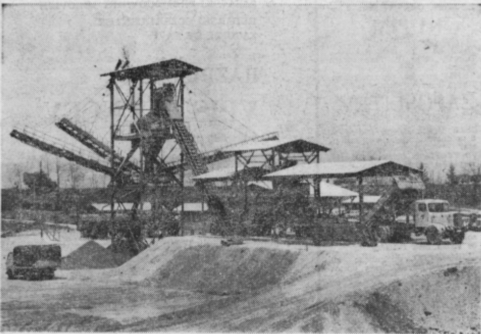
Separacija in drobilnica peska v Krškem, za katero je trboveljska strojna tovarna izdelala in montirala celotno opremo za drobljenje in sejanje peska.
