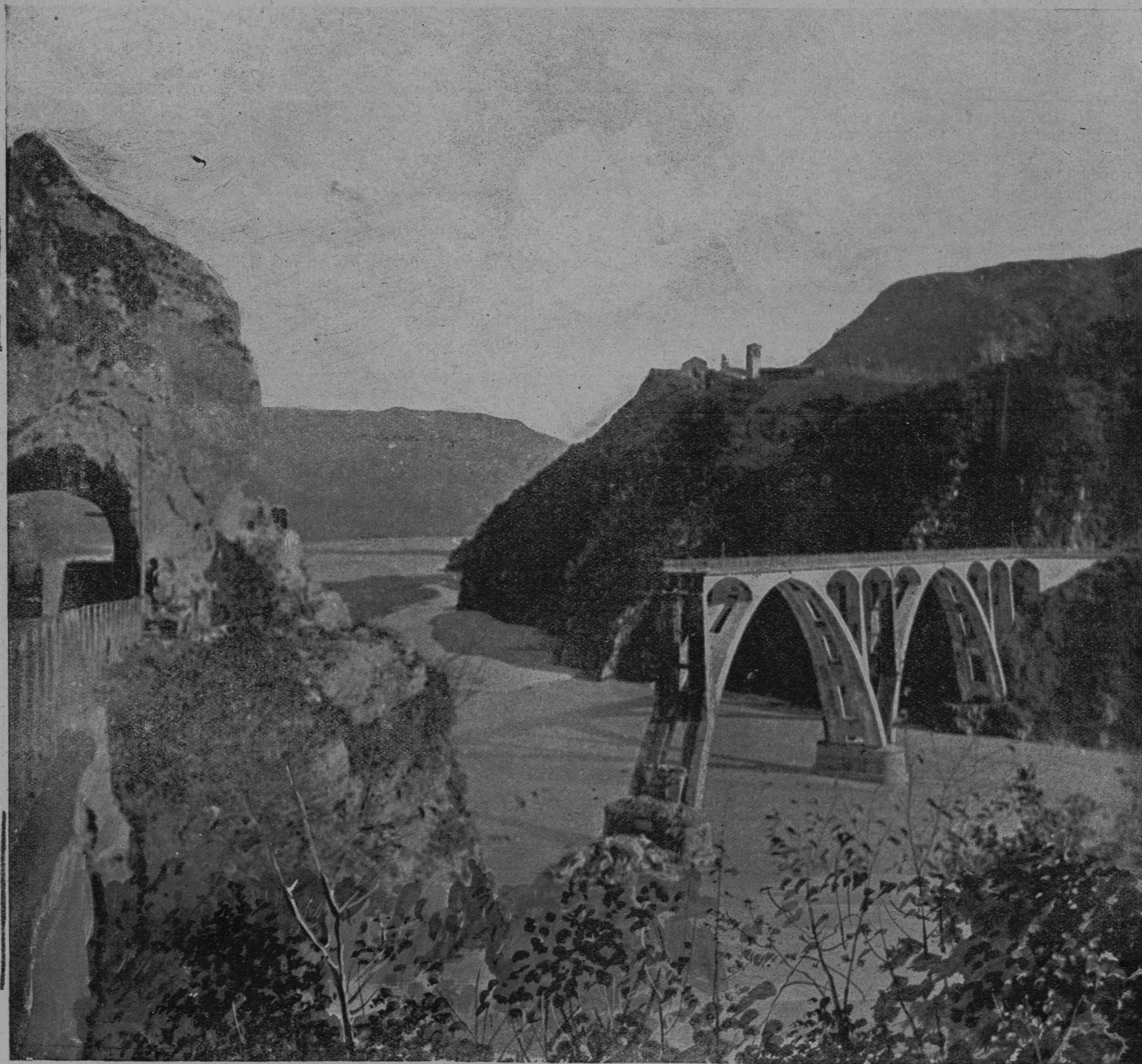
Veliki železniški most čez reko Tilment (Tagliamento) pri S. Danielu v Benečiji, porušen in odrezan od železniških predorov.
