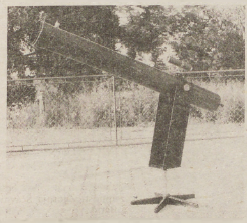
Teleskop s premerom 14 cm in središčno razdaljo 150 cm, ki ga je Tone izdelal sam in zdaj z njim »potuje« od zvezde do zvezde.
