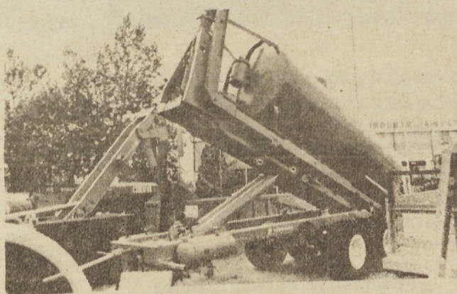
Cisterna z depozitorjem na univerzalnem podvozju
