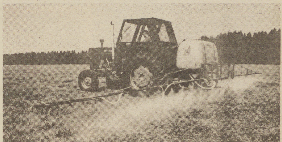
Traktor IMT Beograd z nošeno traktorsko škropilnico Agromehanike.
