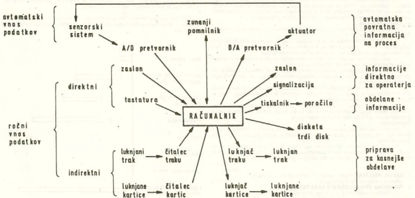
Slika: Možne alternative za računalniško podprt sistem za kontrolo kvalitete
