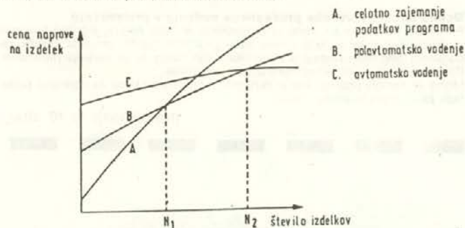
Slika: Stroški stopnje avtomatizacije v odvisnosti od števila končnih izdelkov
